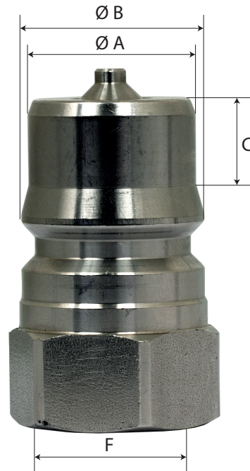
ISO 7241 B
